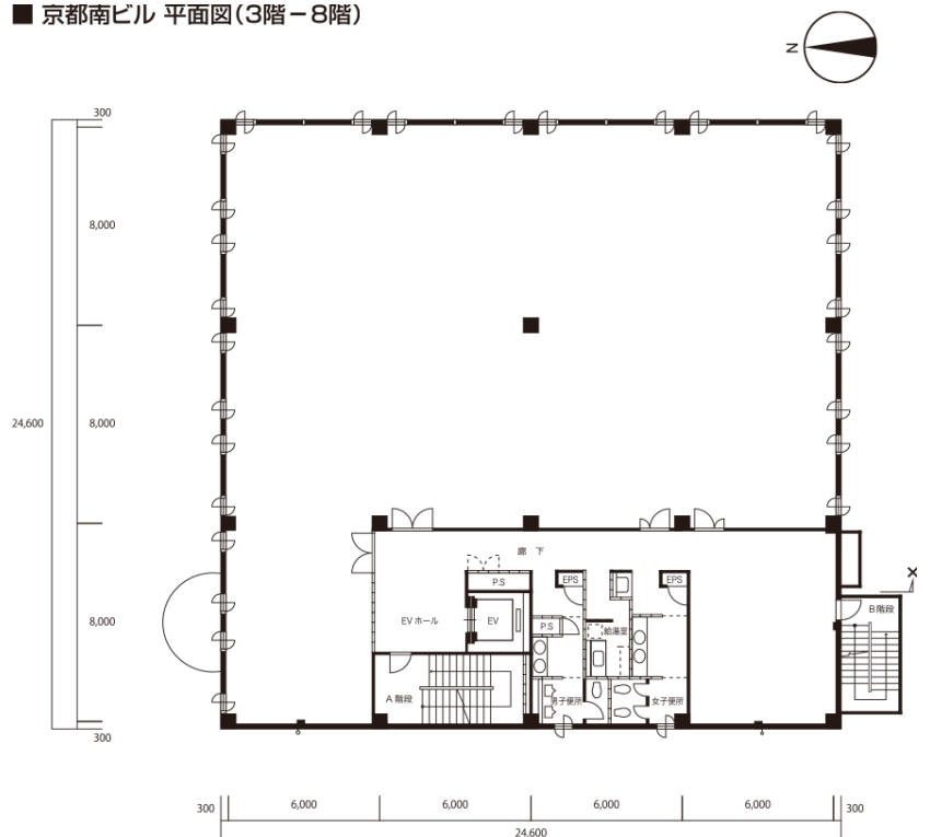
■ 京都南ビル 平面図(3階-8階)
